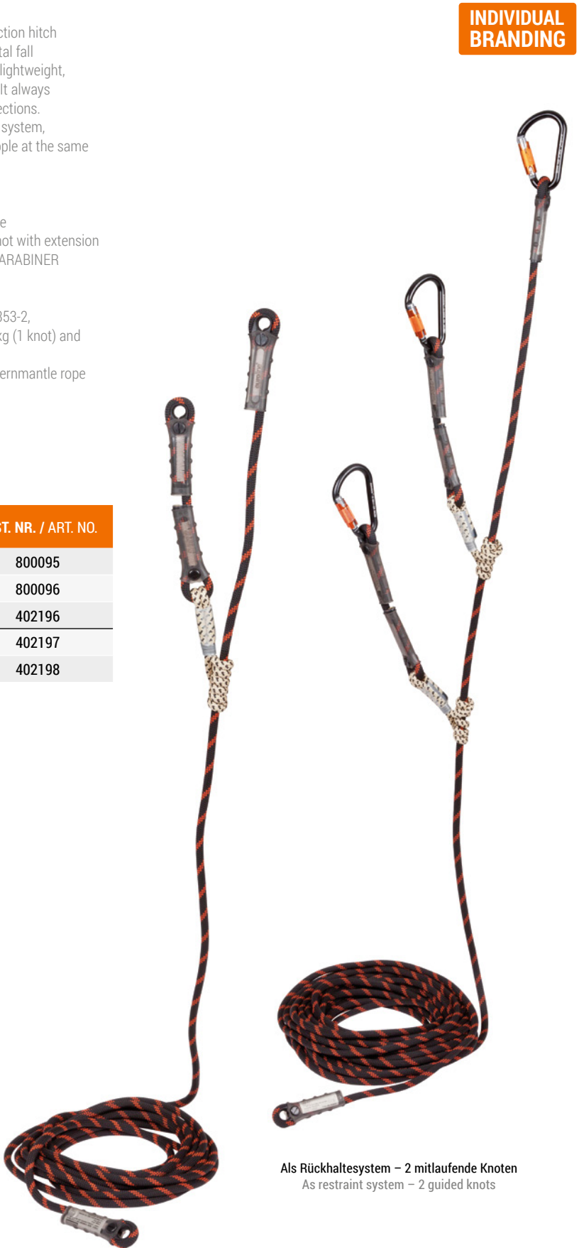
Als Auffangsystem – 1 mitlaufender Knoten As fall arrest system – 1 guided knot
